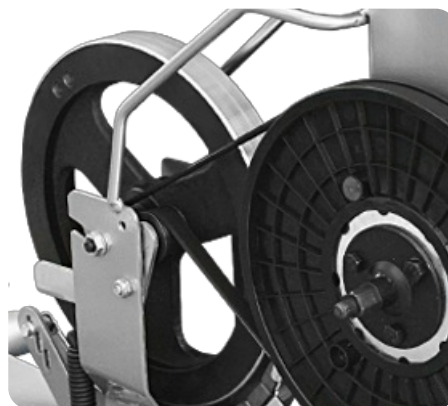
Элементы электромагнитной приводной системы magicFLOW™
